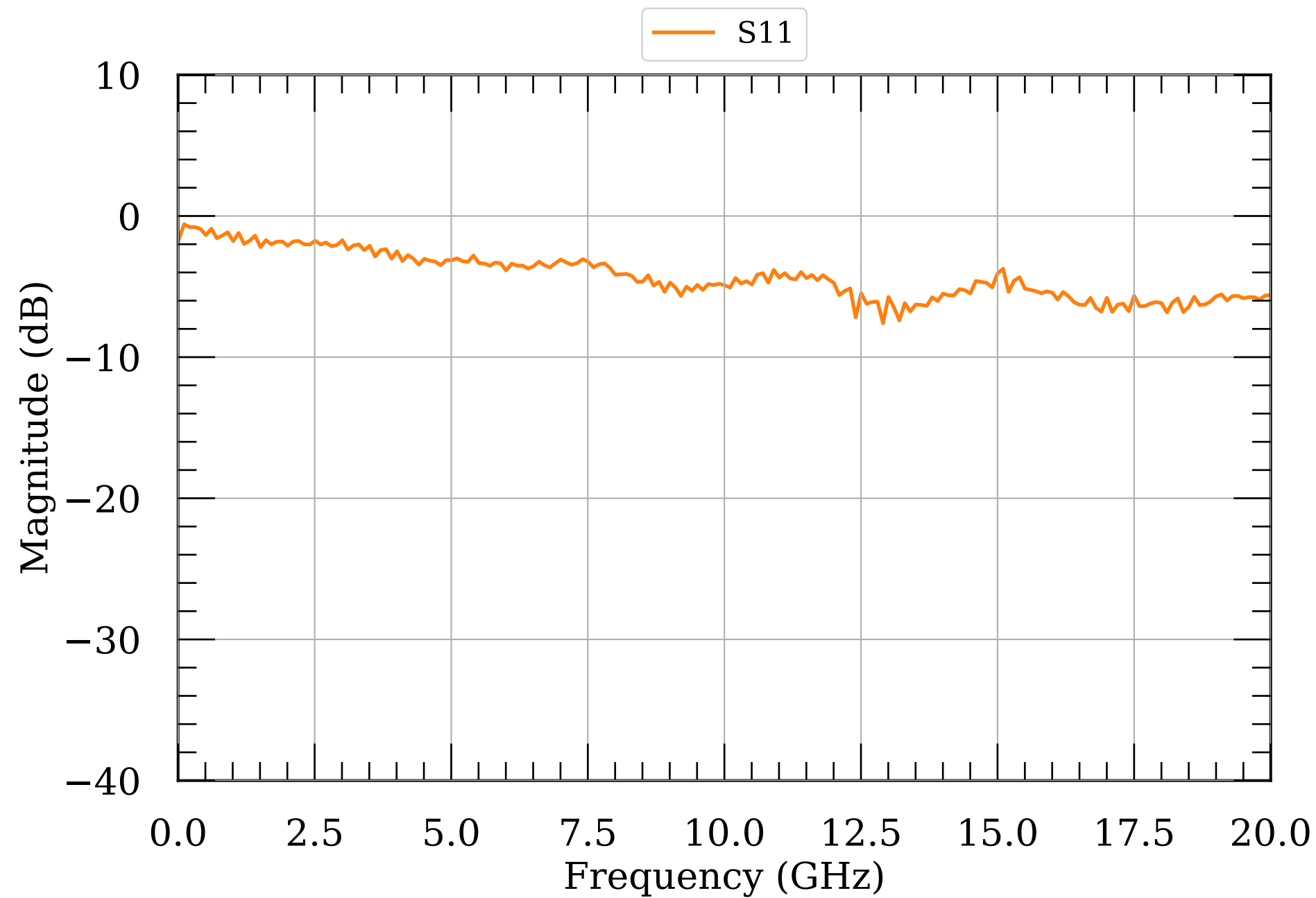
LNA S-params module066
